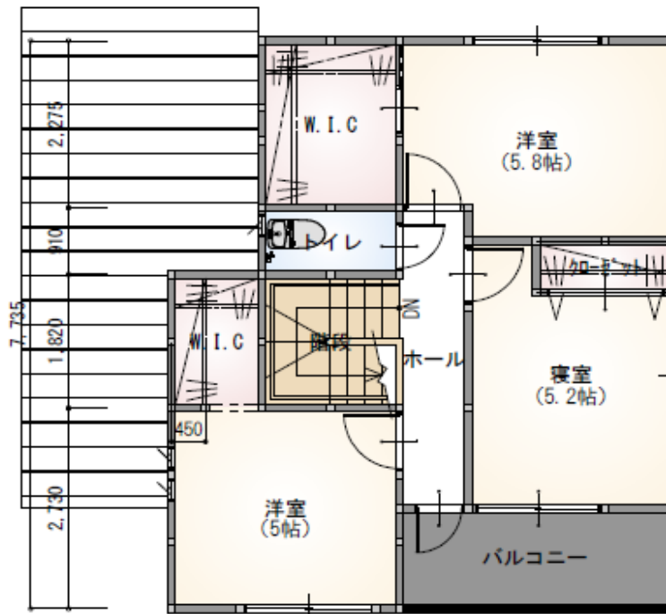
2F 平面図
