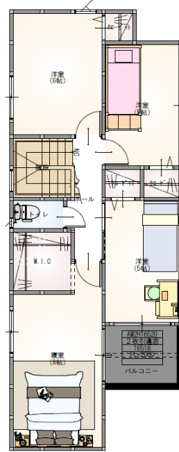
2F 平面図
