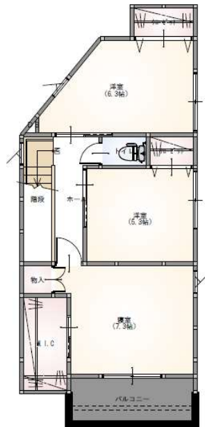
2F 平面図
