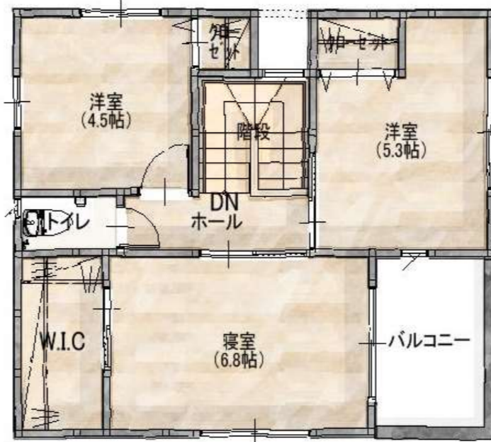
2F 平面図
