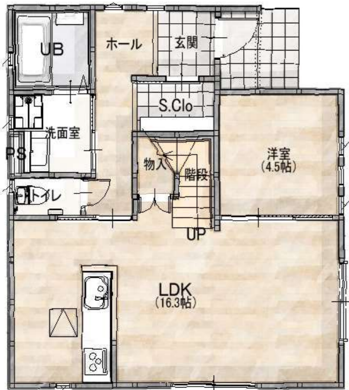
1F 平面図
