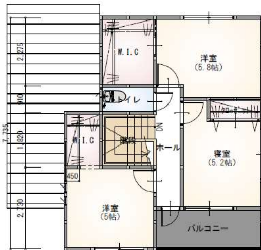
2F 平面図
